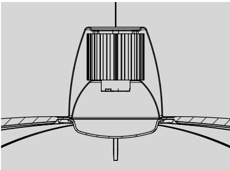
LAMPADA CON DIFFUSORE (A) LAMP WITH DIFFUSER
